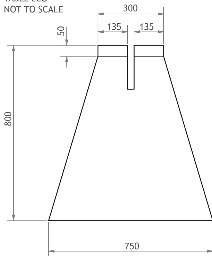
ELEVATION
